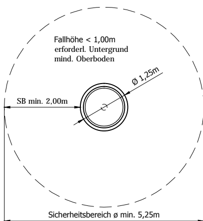
Draufsicht mit Sicherheitsbereich -M. 1:100-
